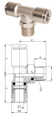
INOXMT: Racor Inst. INOX "T" Orientable Cónica
